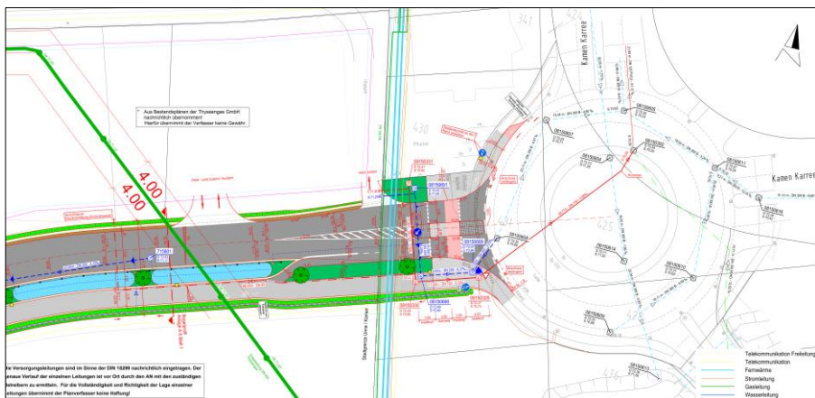
Abbildung 2 Anbindung an bestehenden Kreisverkehrsplatz
